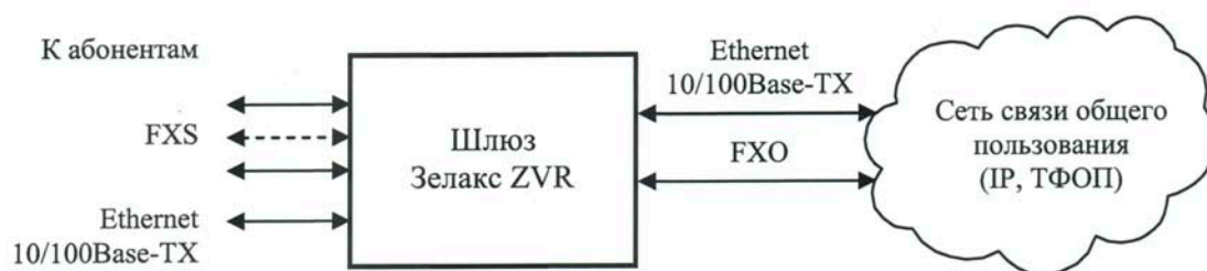
Схема подключения оборудования к сети связи общего пользования
