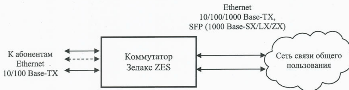
Схема подключения оборудования к сети связи общего пользования
