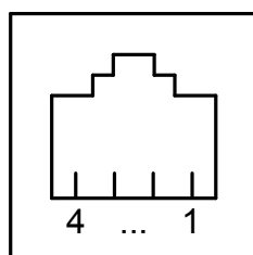
Розетка RJ-11
