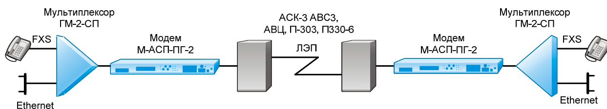
Рис. 3. Организации передачи речевых каналов и подключения к локальной сети с помощью комплекса К-ЛЭП
