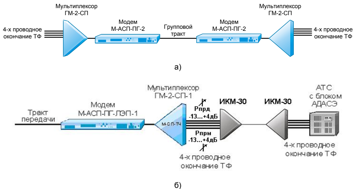
Рис. 9. Организация связи между 4-проводными окончаниями ( а – с помощью двух полукомплектов К-ЛЭП, б – между ГМ-2-СП-1 и окончанием системы передачи - 4-проводный транзит ТФ каналов).
