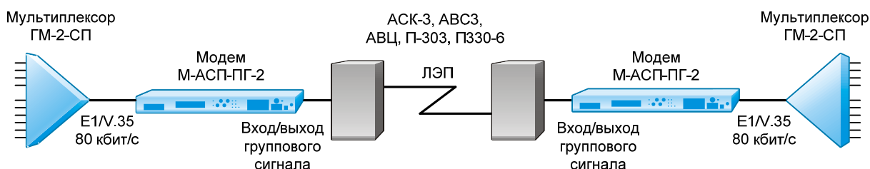
Рис. 1. Подключение модемов М-АСП-ПГ-2 вер. ЛЭП к аппаратуре ВЧ связи для организации цифровой передачи данных и речи по ЛЭП
