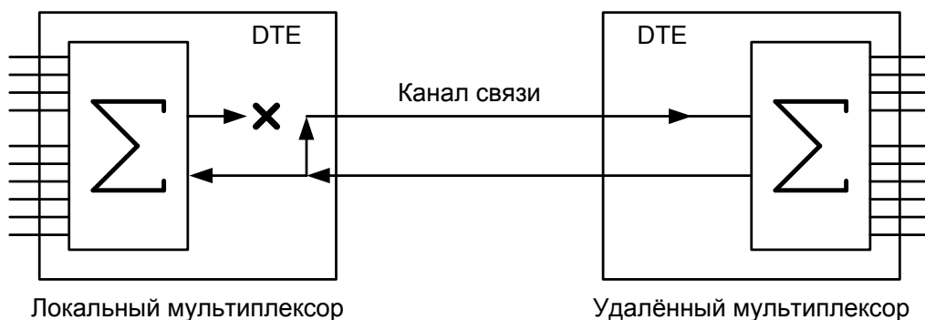
Рис. 10. Проверка в режиме DL — “цифровой шлейф”
