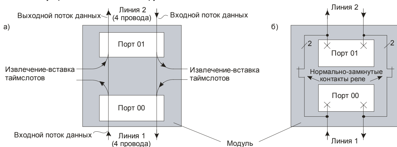
Рис. 4. Передача потоков данных через модули MIM-2xE1A-R и MIME-2xE05-R: а – штатный режим; б – нештатный режим
