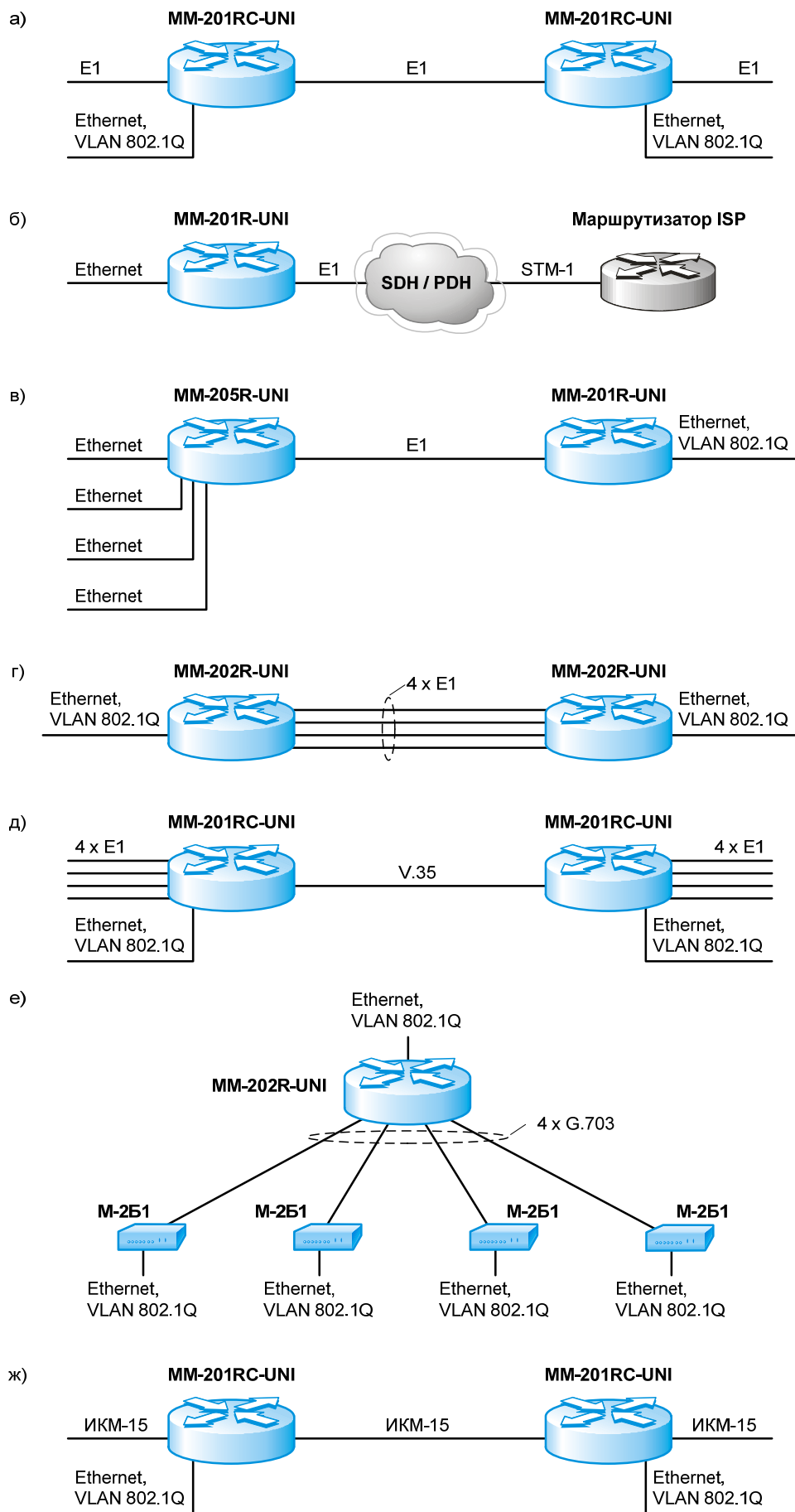
Рис. 2. Примеры использования модулей совместно с устройствами MM-20x
