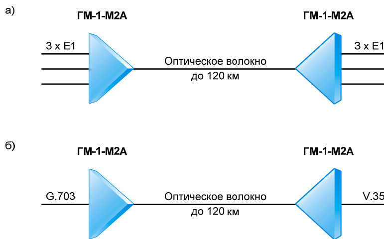
Рис. 1. Примеры использования модулей совместно с мультиплексорами ГМ-1-M2А
